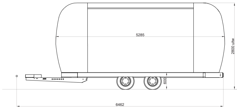
Seitenansicht rechts
